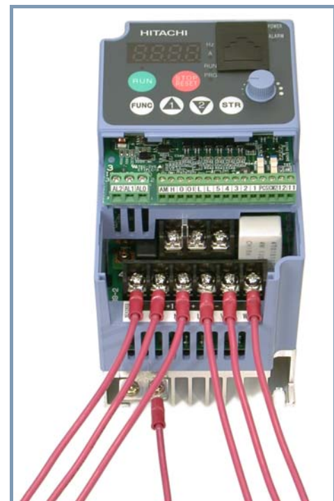
Exemple de câblage L200-037LFU
