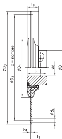
BoWex® FLE-PAC – Dimensions selon SAE
