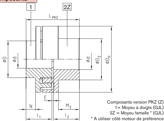
Version PKZ (Z) – (Taille 8 à 30)
