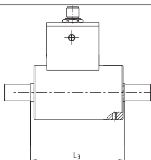
DATAFLEX® 16
