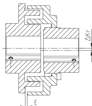
Désalignement radial
