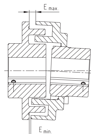
Désalignement angulaire
