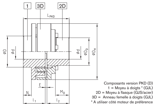
Version PKD (D) – (Taille 15 à 40)
