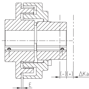
Désalignement axial
