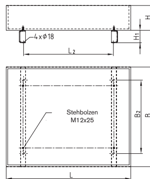
Bac de rétention avec pieds
