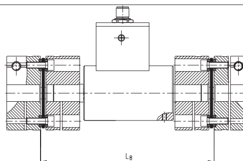
Combinaison DATAFLEX® 16 et RADEX®-NC
