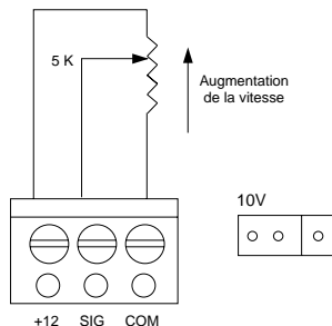
Consigne potentiométrique
