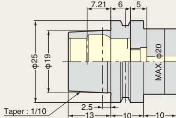
HSK25E DIN69893-5
