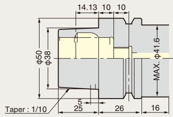
HSK50E DIN69893-5
