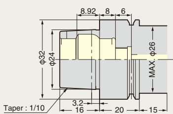
HSK32E DIN69893-5
