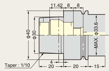
HSK40E DIN69893-5
