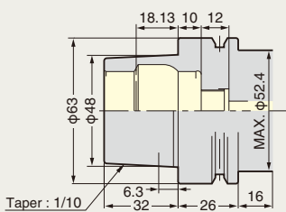
HSK63E DIN69893-5
