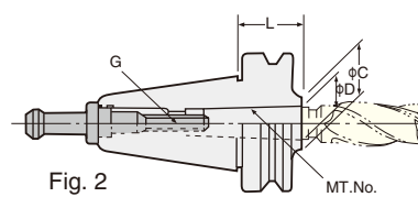
Pull stud draw bolt type.
