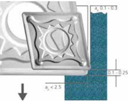
Préréglage des deux coupes du RFP Presetting of roughing and finishing cutting edge
