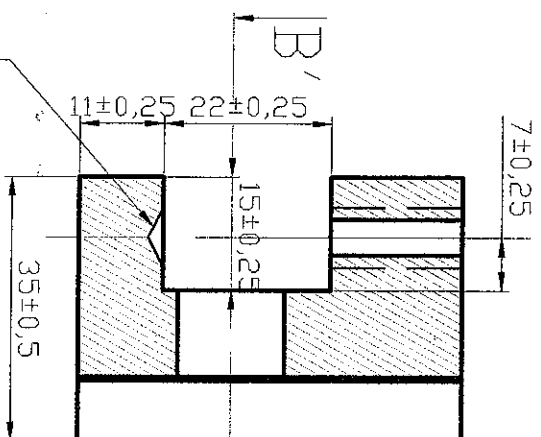
PORTE OUTIL SERONA 900-TS
