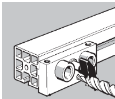
Gabarit de perçage pour foret étagé
