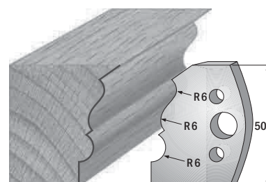
Paar Profilmesser/paire couteaux profilés 690.509 Paar Abweiser/paire limiteurs 691.509
