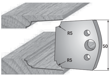
Paar Profilmesser/paire couteaux profilés 690.579 Paar Abweiser/paire limiteurs 691.579
