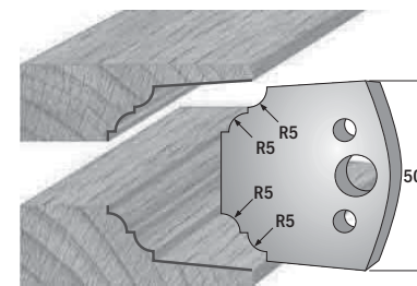
Paar Profilmesser/paire couteaux profilés 690.580 Paar Abweiser/paire limiteurs 691.580
