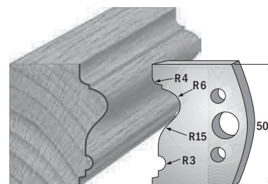
Paar Profilmesser/paire couteaux profilés 690.512 Paar Abweiser/paire limiteurs 691.512
