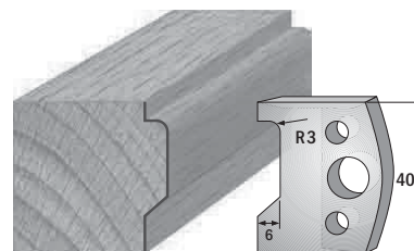
Paar Profilmesser/paire couteaux profilés 690.032 Paar Abweiser/paire limiteurs 691.032
