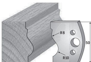
Paar Profilmesser/paire couteaux profilés 690.510 Paar Abweiser/paire limiteurs 691.510
