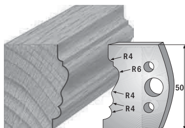
Paar Profilmesser/paire couteaux profilés 690.511 Paar Abweiser/paire limiteurs 691.511
