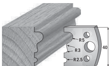
Paar Profilmesser/paire couteaux profilés 690.033 Paar Abweiser/paire limiteurs 691.033
