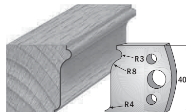
Paar Profilmesser/paire couteaux profilés 690.110 Paar Abweiser/paire limiteurs 691.110
