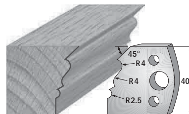
Paar Profilmesser/paire couteaux profilés 690.107 Paar Abweiser/paire limiteurs 691.107
