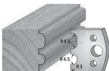
Paar Profilmesser/paire couteaux profilés 690.007 Paar Abweiser/paire limiteurs 691.007
