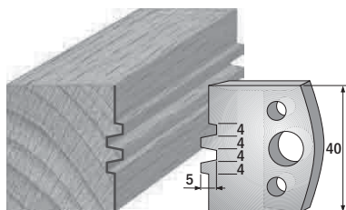
Paar Profilmesser/paire couteaux profilés 690.075 Paar Abweiser/paire limiteurs 691.075
