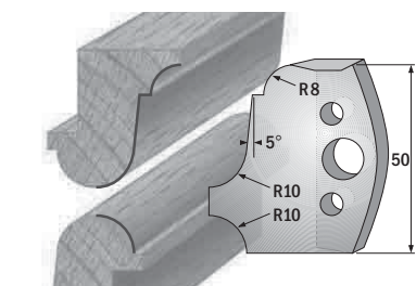
Paar Profilmesser/paire couteaux profilés 690.557 Paar Abweiser/paire limiteurs 691.557
