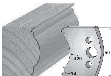
Paar Profilmesser/paire couteaux profilés 690.507 Paar Abweiser/paire limiteurs 691.507
