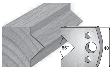
Paar Profilmesser/paire couteaux profilés 690.034 Paar Abweiser/paire limiteurs 691.034
