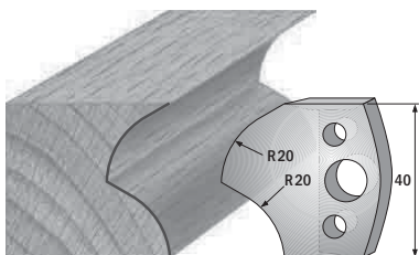
Paar Profilmesser/paire couteaux profilés 690.120 Paar Abweiser/paire limiteurs 691.120
