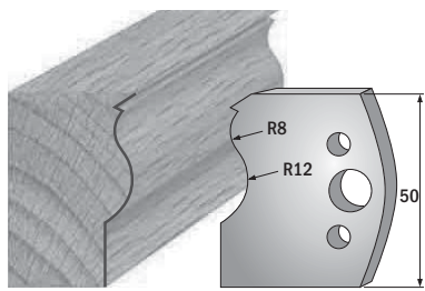
Paar Profilmesser/paire couteaux profilés 690.578 Paar Abweiser/paire limiteurs 691.578
