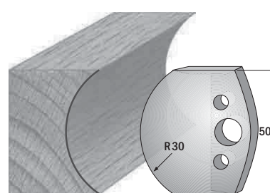
Paar Profilmesser/paire couteaux profilés 690.544 Paar Abweiser/paire limiteurs 691.544
