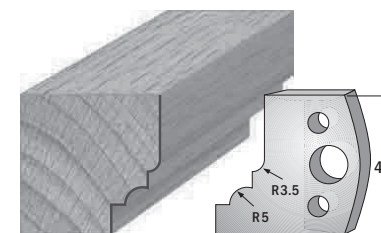
Paar Profilmesser/paire couteaux profilés 690.020 Paar Abweiser/paire limiteurs 691.020
